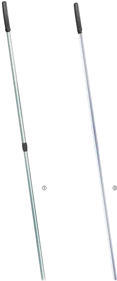
① VERMOP® Teleskopstiel Am Griff verstellbar Länge: Von 90 bis 165 cm 3210022 42,90 €
